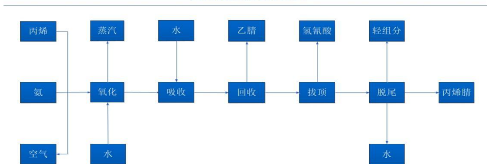
丙烯腈工艺流程图
