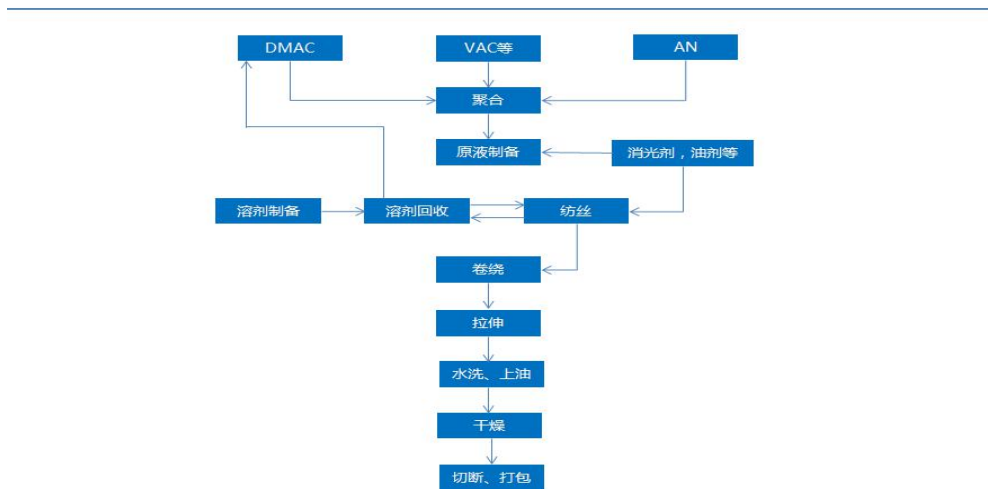
腈纶DMAC湿法二步法工艺图
