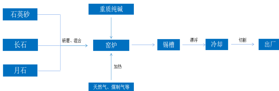
平板玻璃工艺流程图
