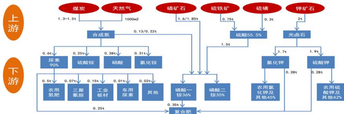
化肥产业链流程图
