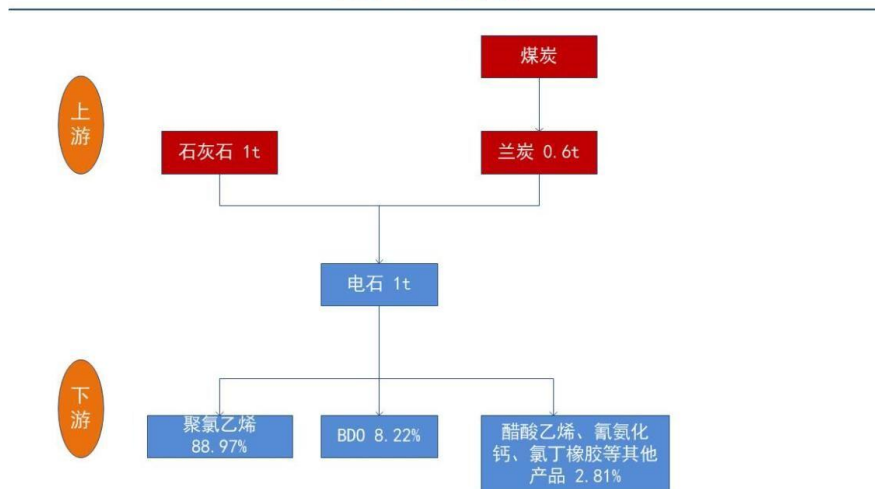
电石产业链流程图
