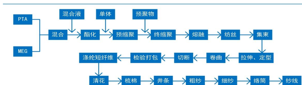
涤纶短纤生产工艺流程图
