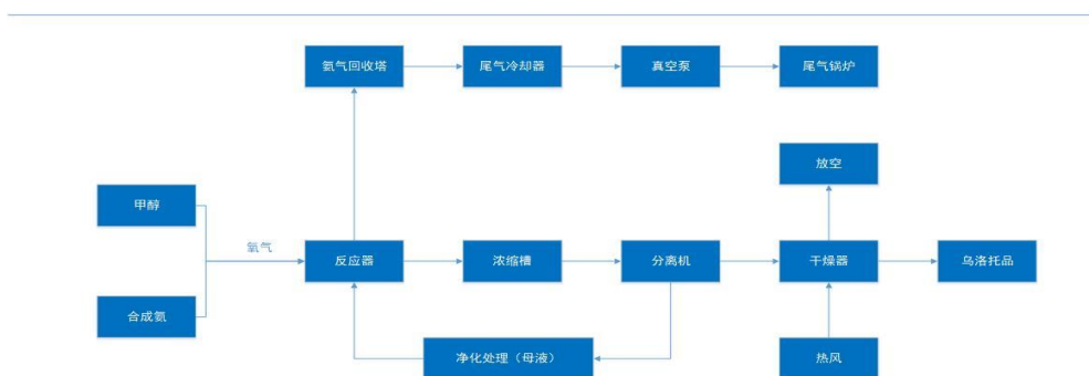
气相法制乌洛托品生产工艺流程图
