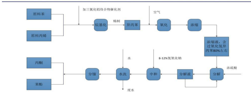
丙酮生产工艺流程图
