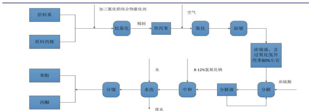
苯酚生产工艺流程图
