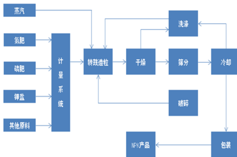
图：转鼓造粒工艺技术
