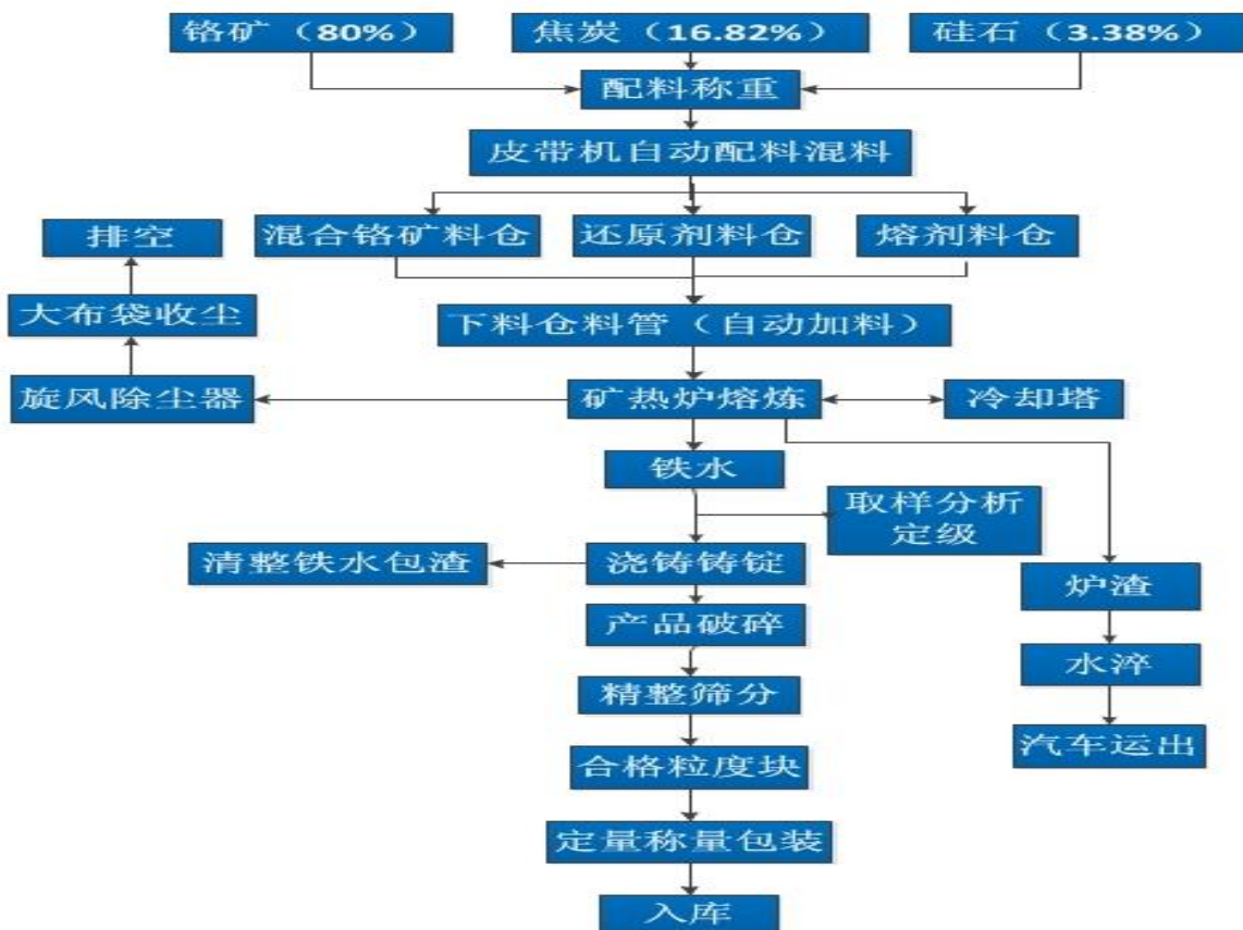
高碳铬铁生产工艺流程图
