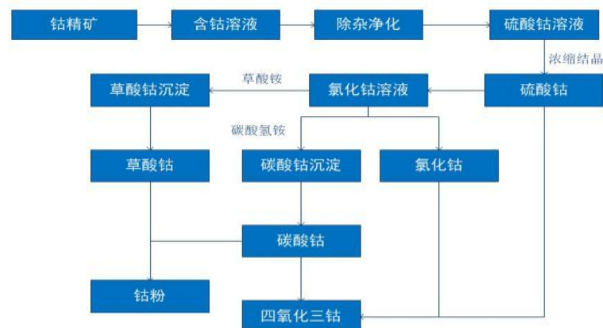
工艺流程图
