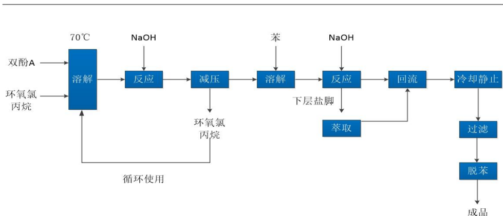
双酚A型环氧树脂生产工艺图
