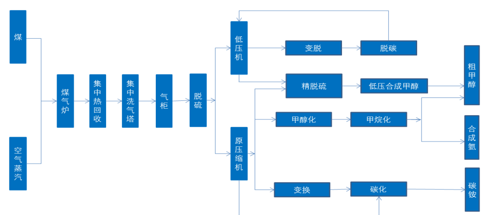
联醇生产工艺流程图
