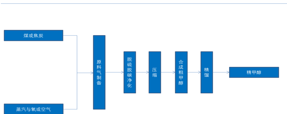
煤制甲醇生产工艺流程图
