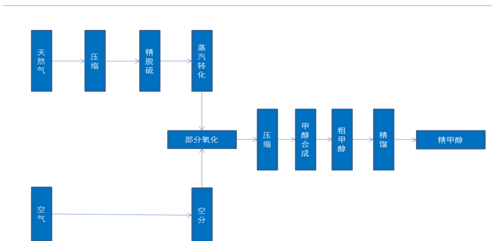
天然气制甲醇生产工艺流程图
