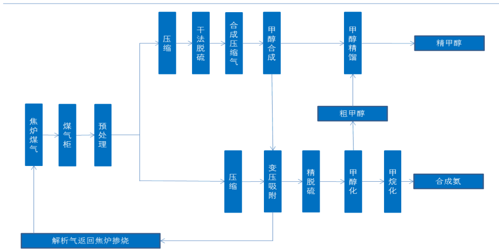
焦炉制甲醇工艺流程图
