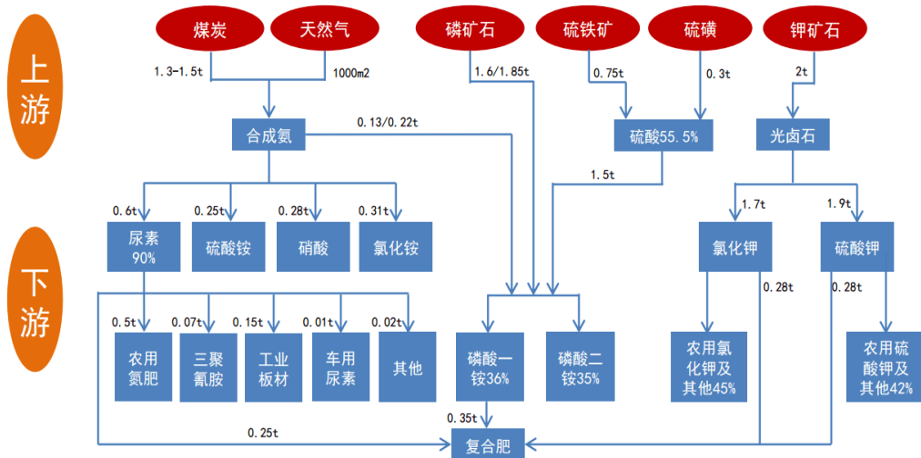
化肥产业链流程图
