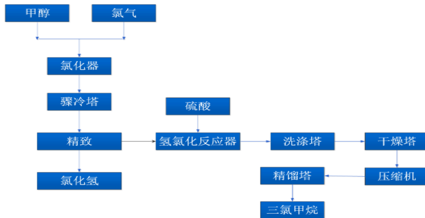
三氯乙烯生产工艺流程图
