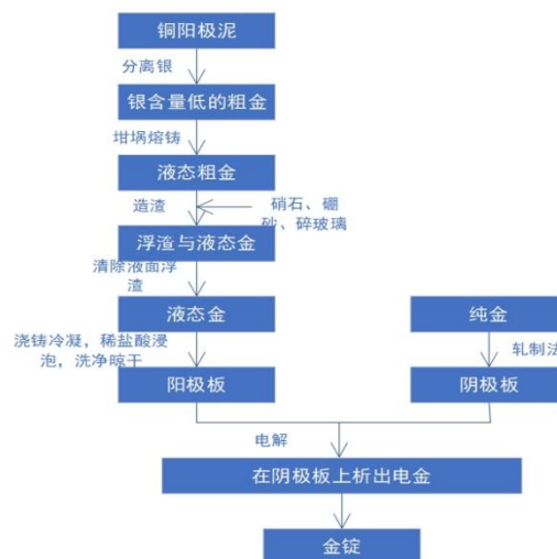
电解法金锭生产工艺流程图
