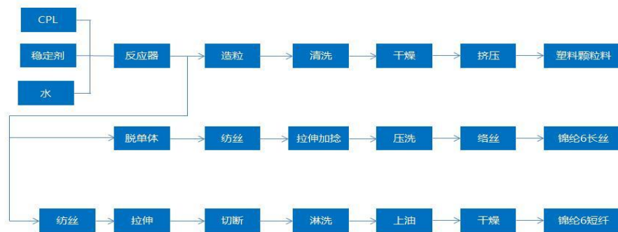
己内酰胺制锦纶6纤维工艺流程图
