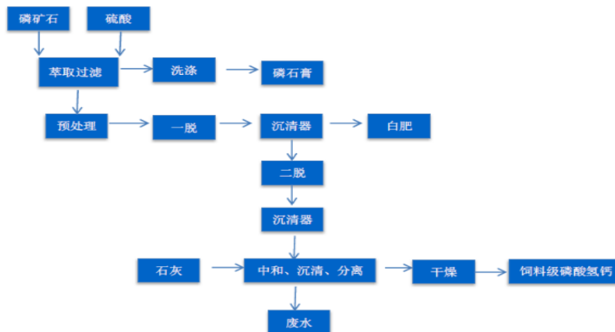
饲料级磷酸氢钙生产工艺流程图
