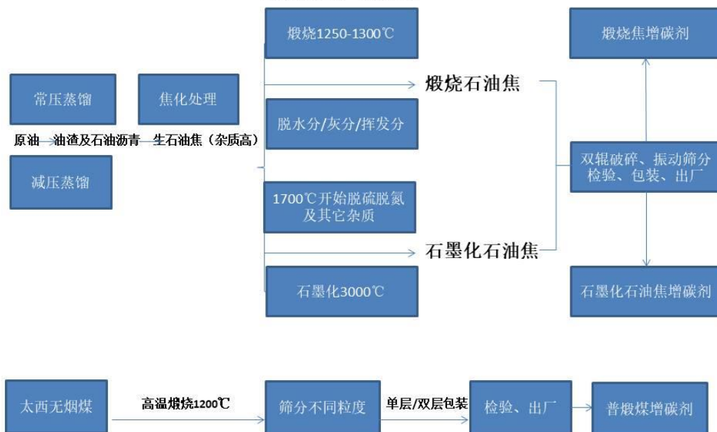
增碳剂生产工艺图
