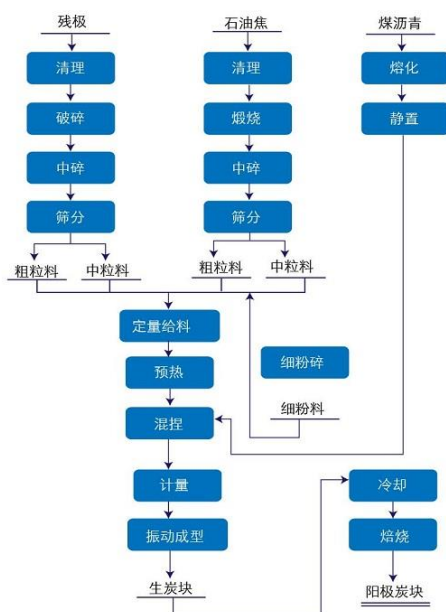
预焙阳极工艺流程图
