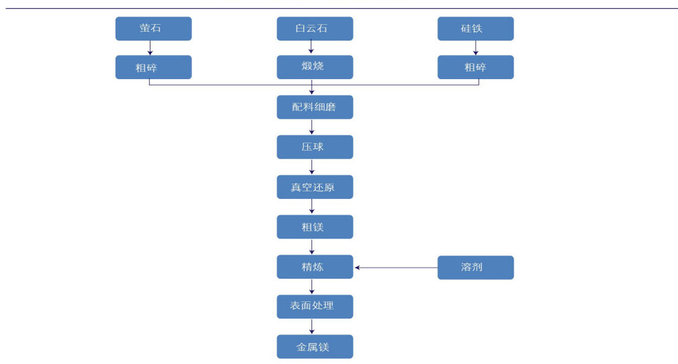
有色—镁生产工艺流程
