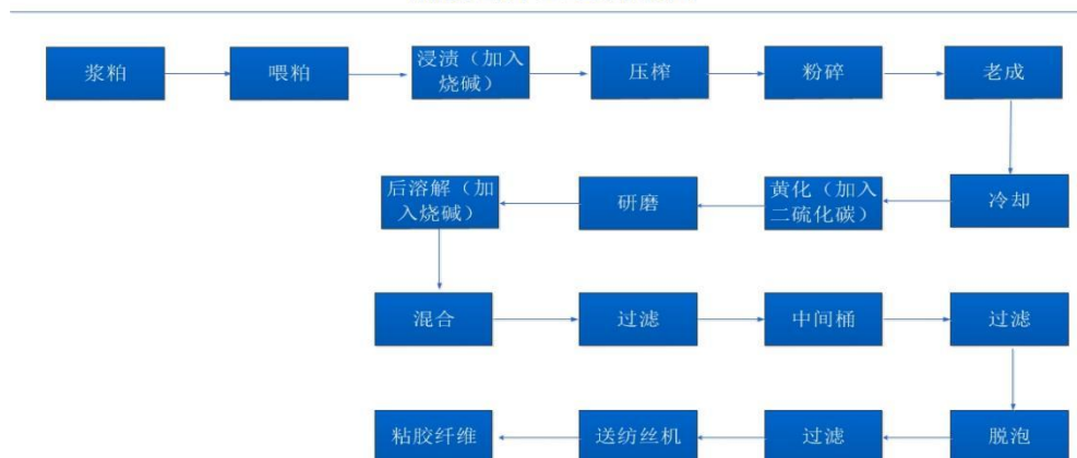
粘胶短纤工艺流程图
