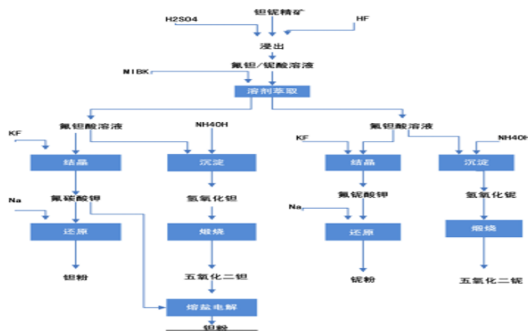
中国铌钽产业链图
