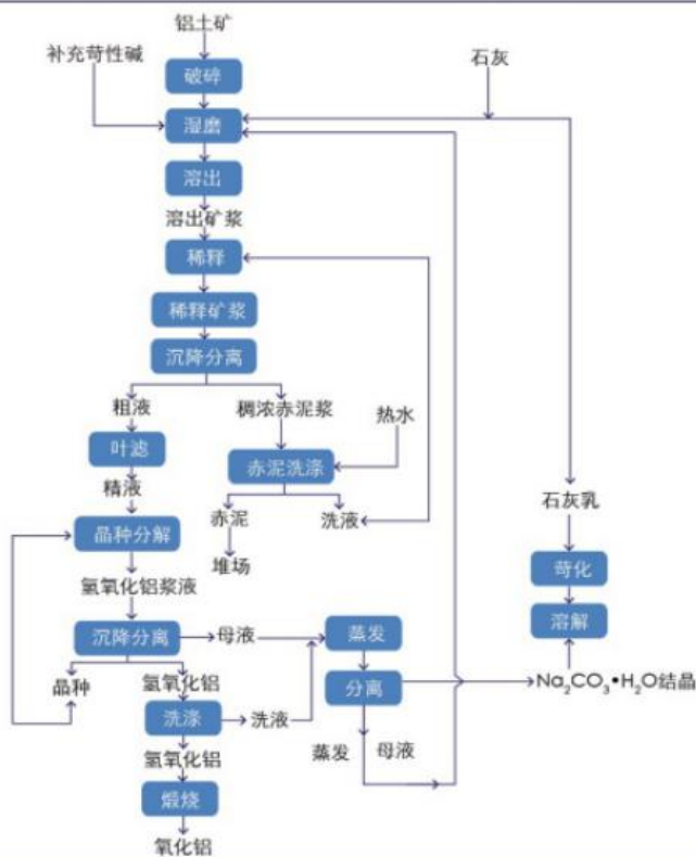
有色— 氢氧化铝生产工艺图
