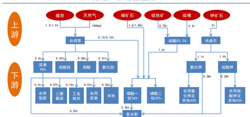
化肥产业链流程图
