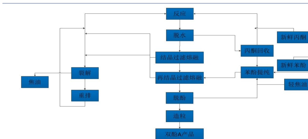
双酚A工艺流程图
