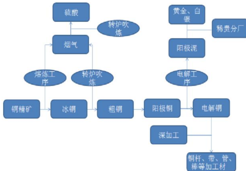
铜火法冶炼工艺流程图
