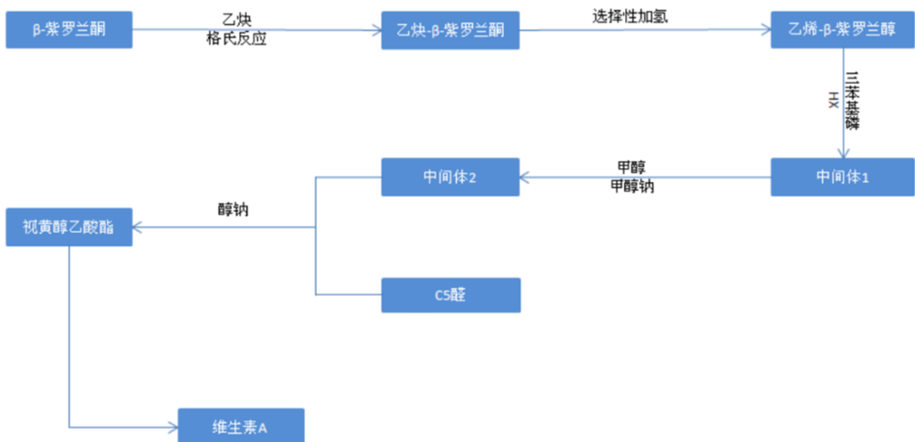
图：维生素 A 生产工艺流程图
