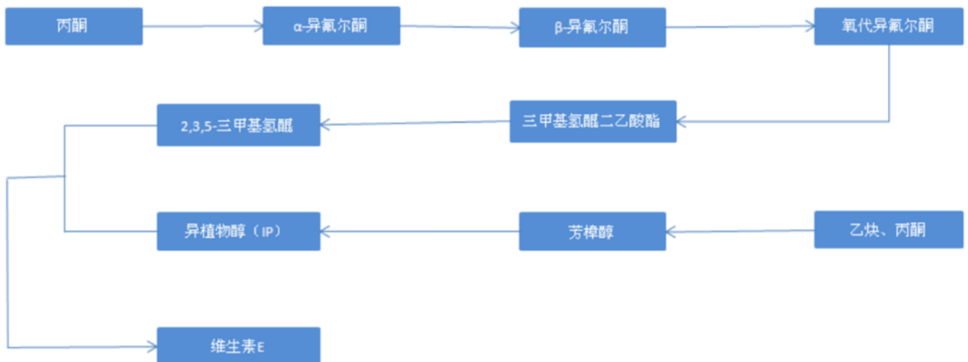
图：维生素 E 生产工艺流程图
