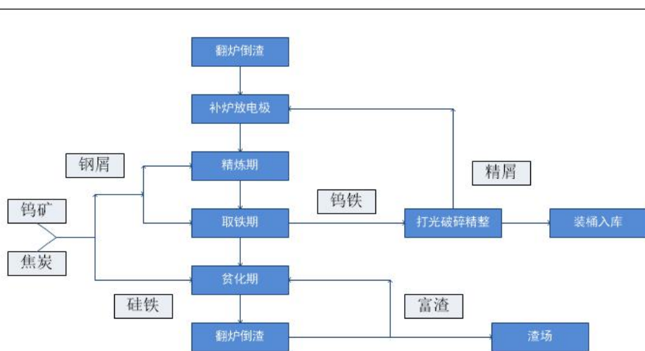
钨铁（取铁法）生产工艺流程图
