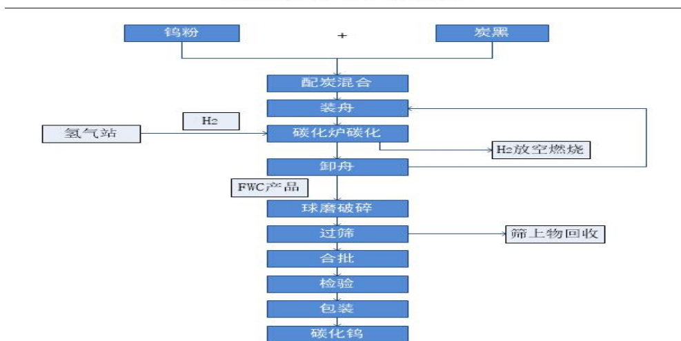
碳化钨生产工艺流程图
