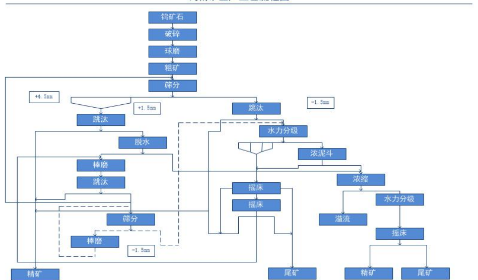
钨精矿生产工艺流程图
