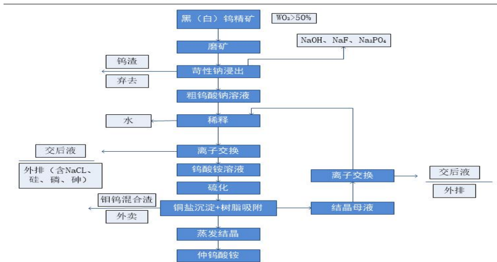
仲钨酸铵生产工艺流程图
