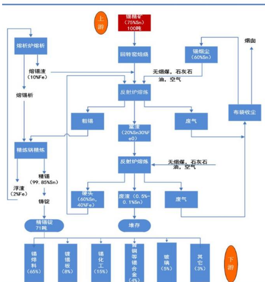
锡生产工艺流程图
