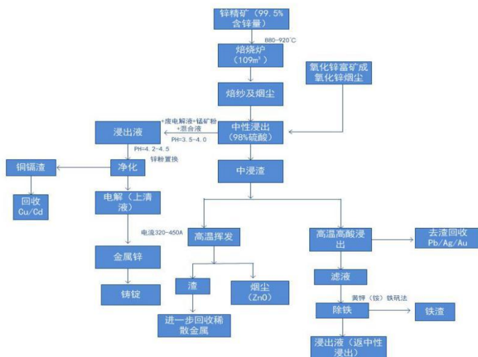
锌冶炼工艺流程图
