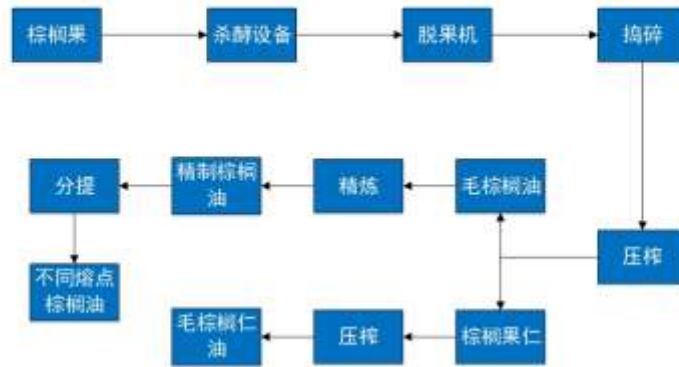
棕榈油压榨法生产工艺图
